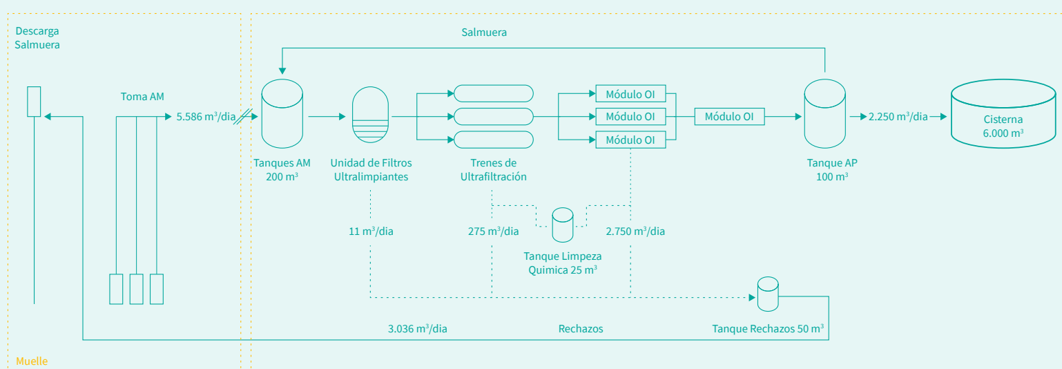
Figura 9 Proceso en una planta desaladora
